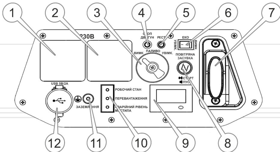
Рисунок 2. Панель керування.
